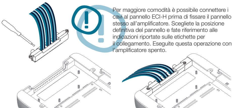
■ Montaggio a filo del pannello
